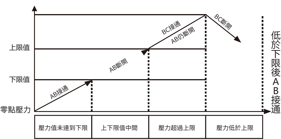
05K電接點功能（壓力電接點）
