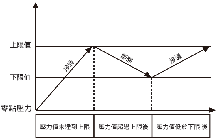
01K壓力開關功能（高停低啟）
