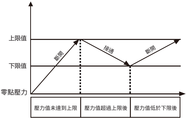
03K壓力開關功能（高啟低停）
